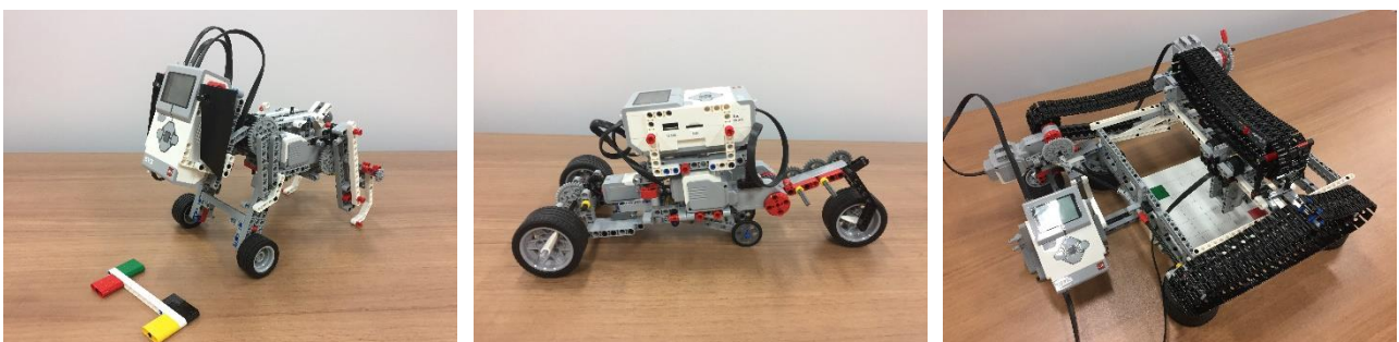
Figure 3 Robots ejemplo para estudiantes y DEMOS
